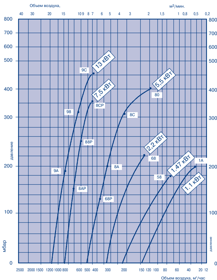
Диаграмма для выбора компрессора, трехфазный двигатель, 50 Гц
